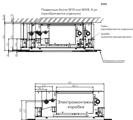
Внутренний блок и воздушная панель
