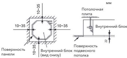
(а) Потолочный монтаж спanelью
